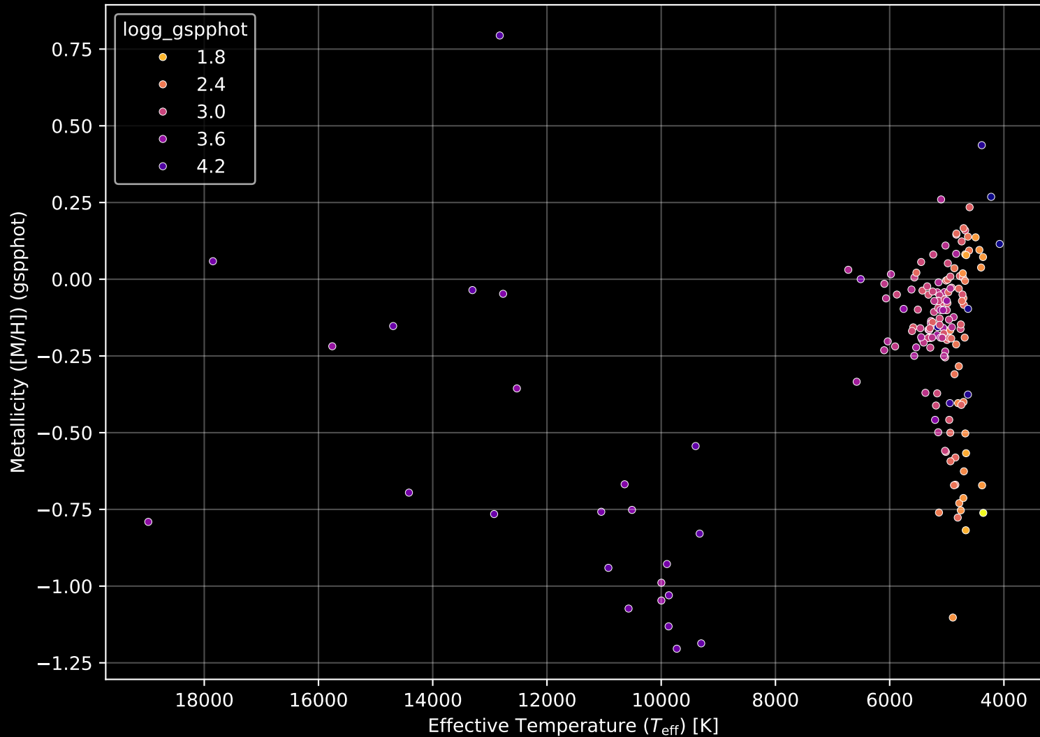
APOGEE DR17 Field: [218-04] Stellar Population Parameters (n= 176)
